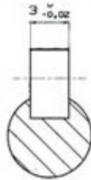
SEZ B-B
